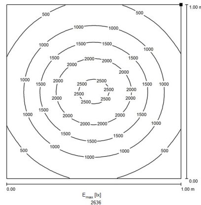
Isoluxdiagramm, Meßabstand 50 cm
